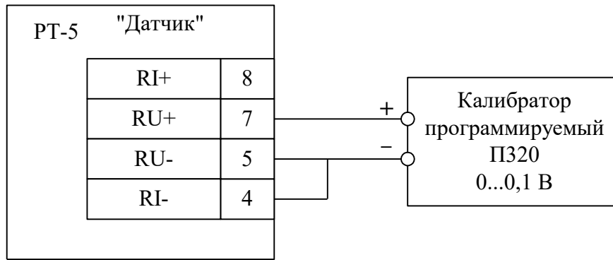
Рисунок 13 - Схема подключения для ввода корректирующего коэффициента и проверки регулятора при работе с преобразователями с выходным напряжением
