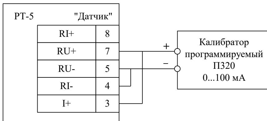
Рисунок 12 - Схема подключения для ввода корректирующего коэффициента и проверки регулятора при работе с преобразователями с выходным током
