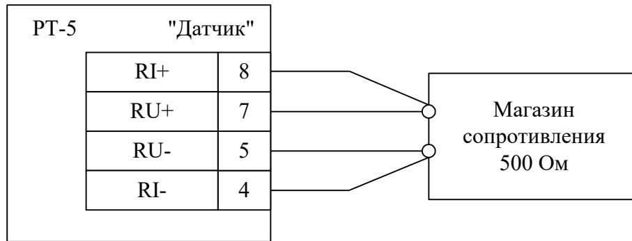
Рисунок 11 - Схема подключения для ввода корректирующего коэффициента и проверки регулятора при работе с ТС
