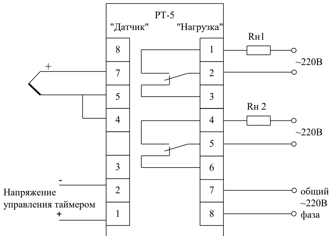
Рисунок 7 - Схема соединений при использовании термопар (ТХА, ТХК, ТЖК, ТНН)
