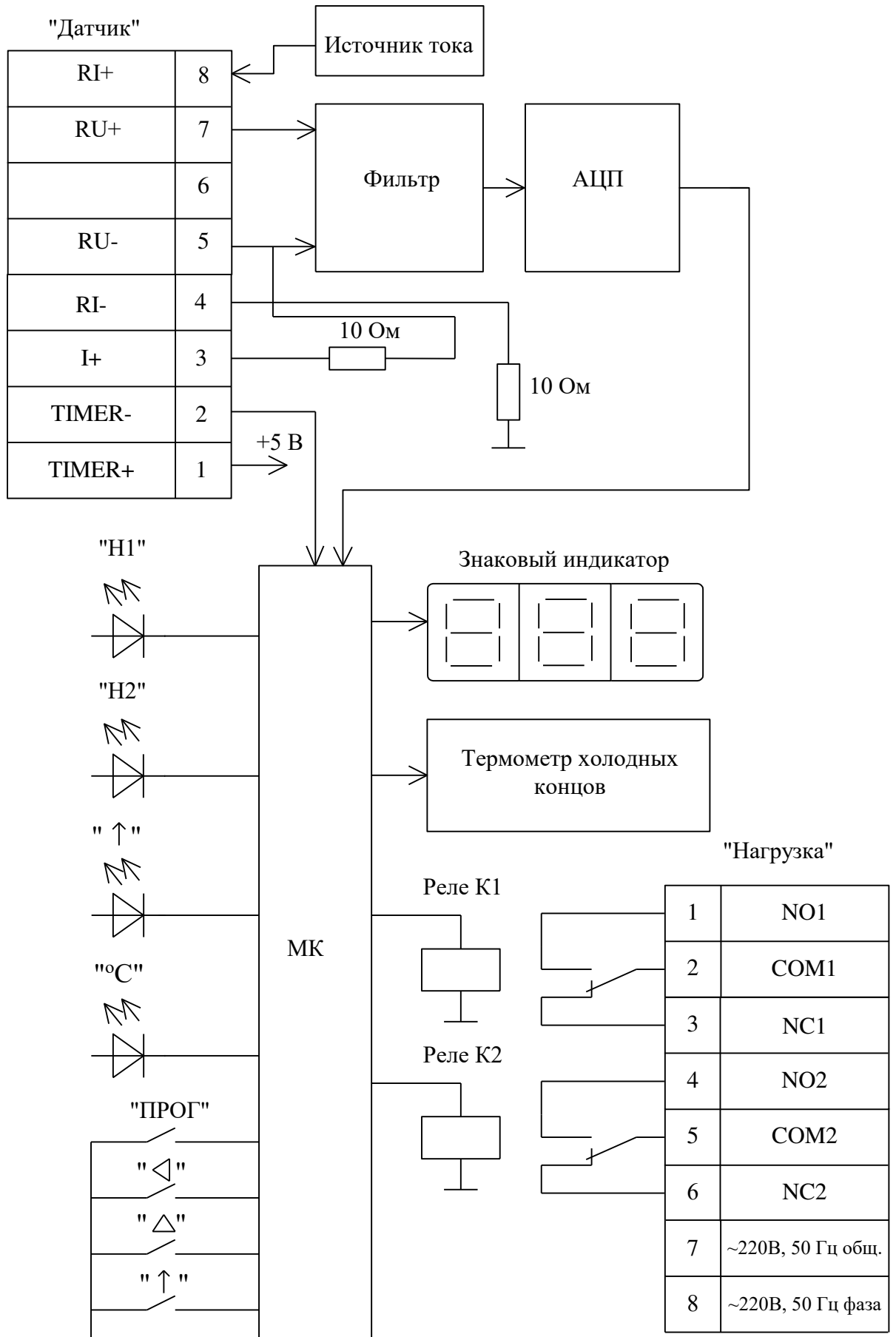
Рисунок 2 - Функциональная схема регулятора
