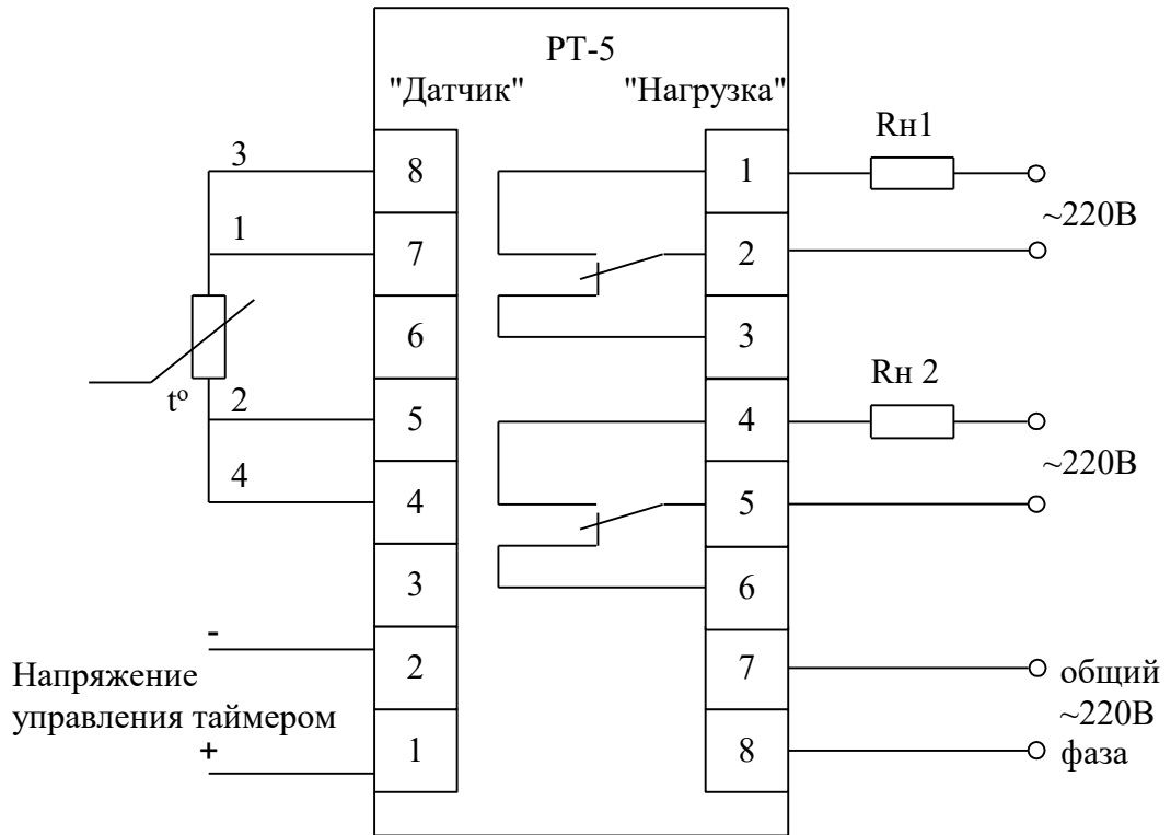
Рисунок 6 - Схема соединений при использовании термопреобразователя сопротивления
