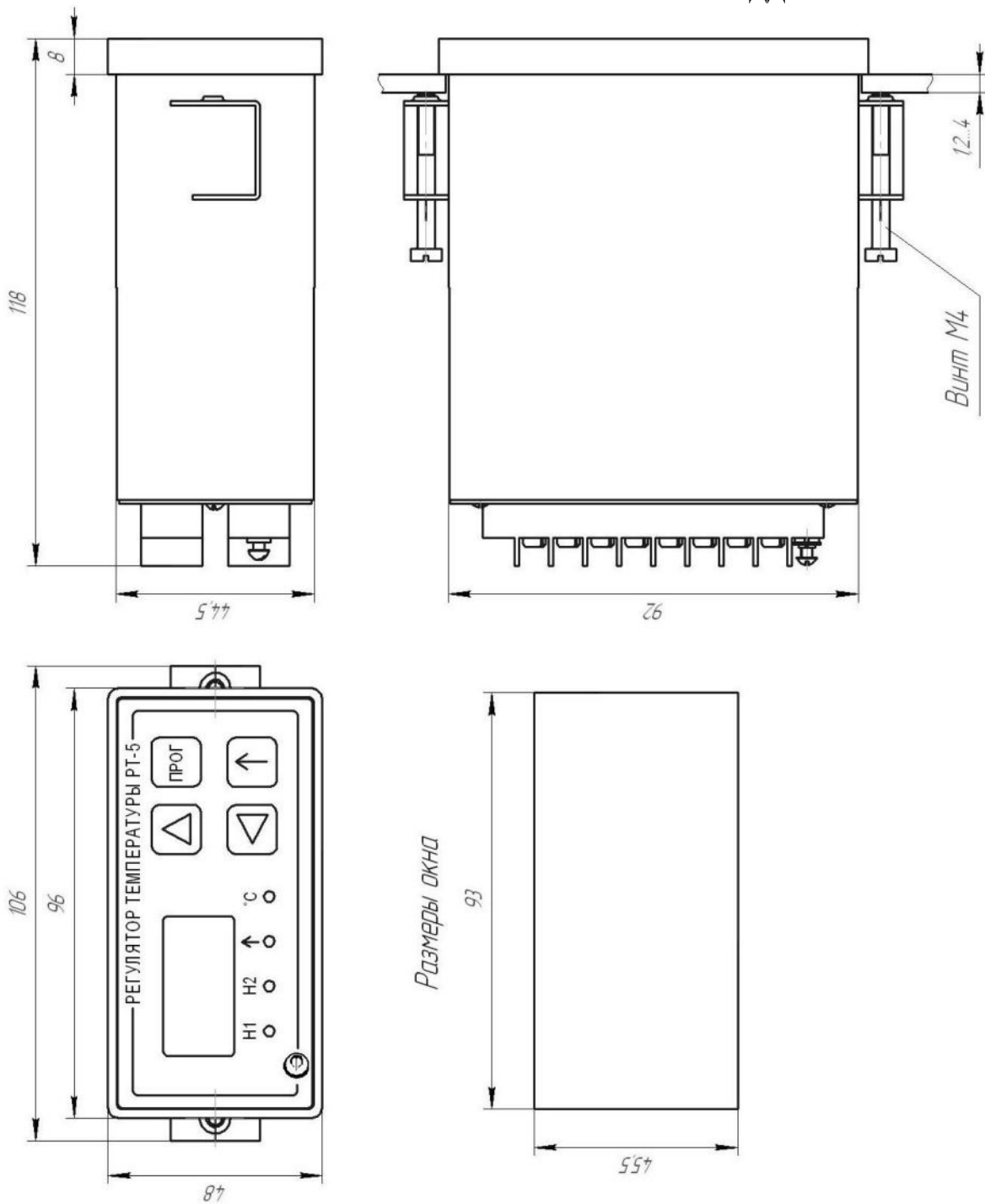
Рисунок 4 – Габаритные и установочные размеры регулятора щитового испол-
